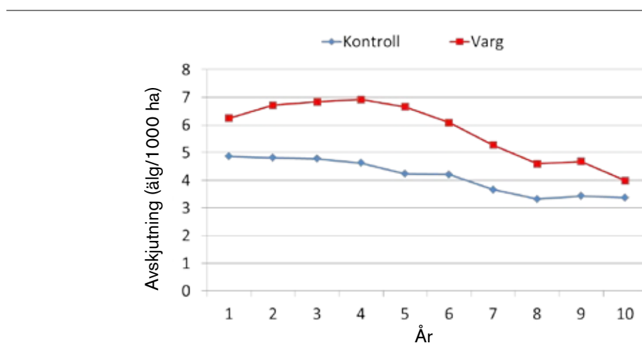
Figur 2. Avskjutningen av älg per 1000 ha i medeltal för 6 områden där vargarna hade haft etablerade revir i minst 10 år (röd linje) och i närliggande kontrollområden utan varg (blå linje).
